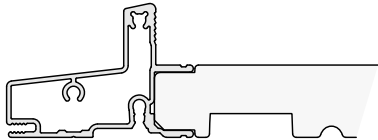
Thin Jamb Cladding - PF2052
