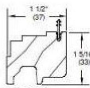
W9787 Head Jamb Stop
