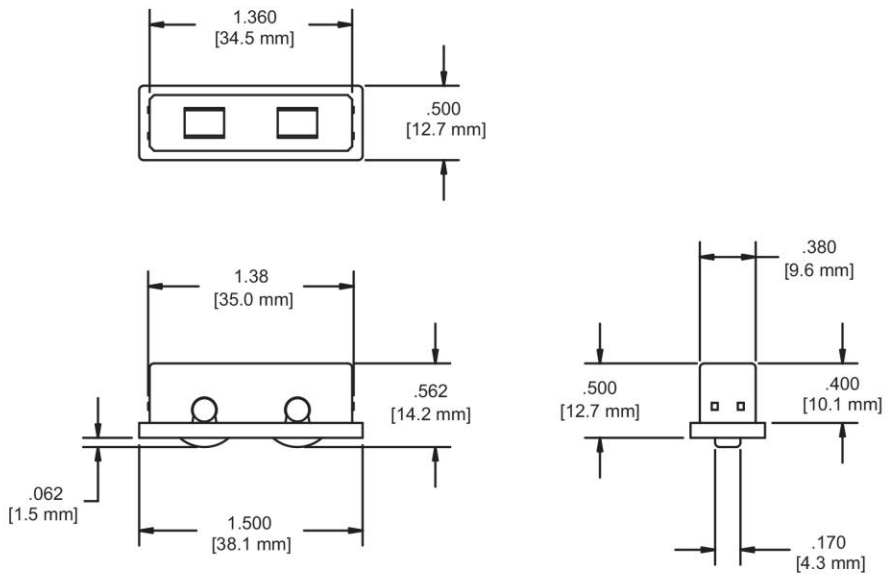
FIG. 2 4231-1000 ROLLER
