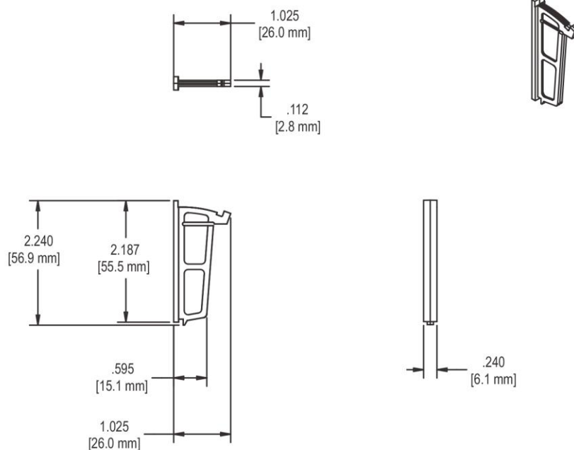
FIG. 1 22833 VENT STOP
