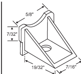
900-5522 Crown
