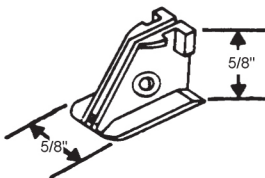
74-503 Keller
